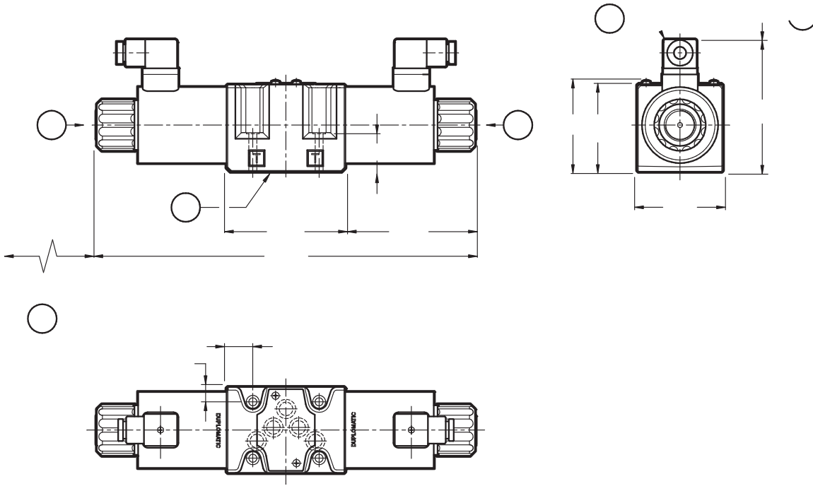
DSE5-A* DSE5-C*
