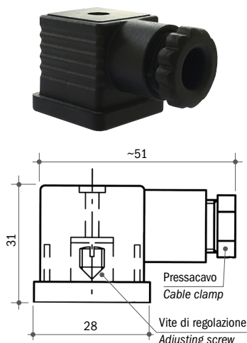
Connettore DIN 40050 DIN 40050 connector
