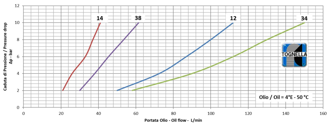
FT 2270/5 PORTATA FLUSSO LIBERO / FREE FLOW
